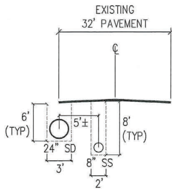
CROSS SECTION 1 VIERA AVE.
