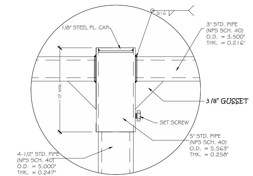
DETAIL A Scale: 1" = 1'-0"
