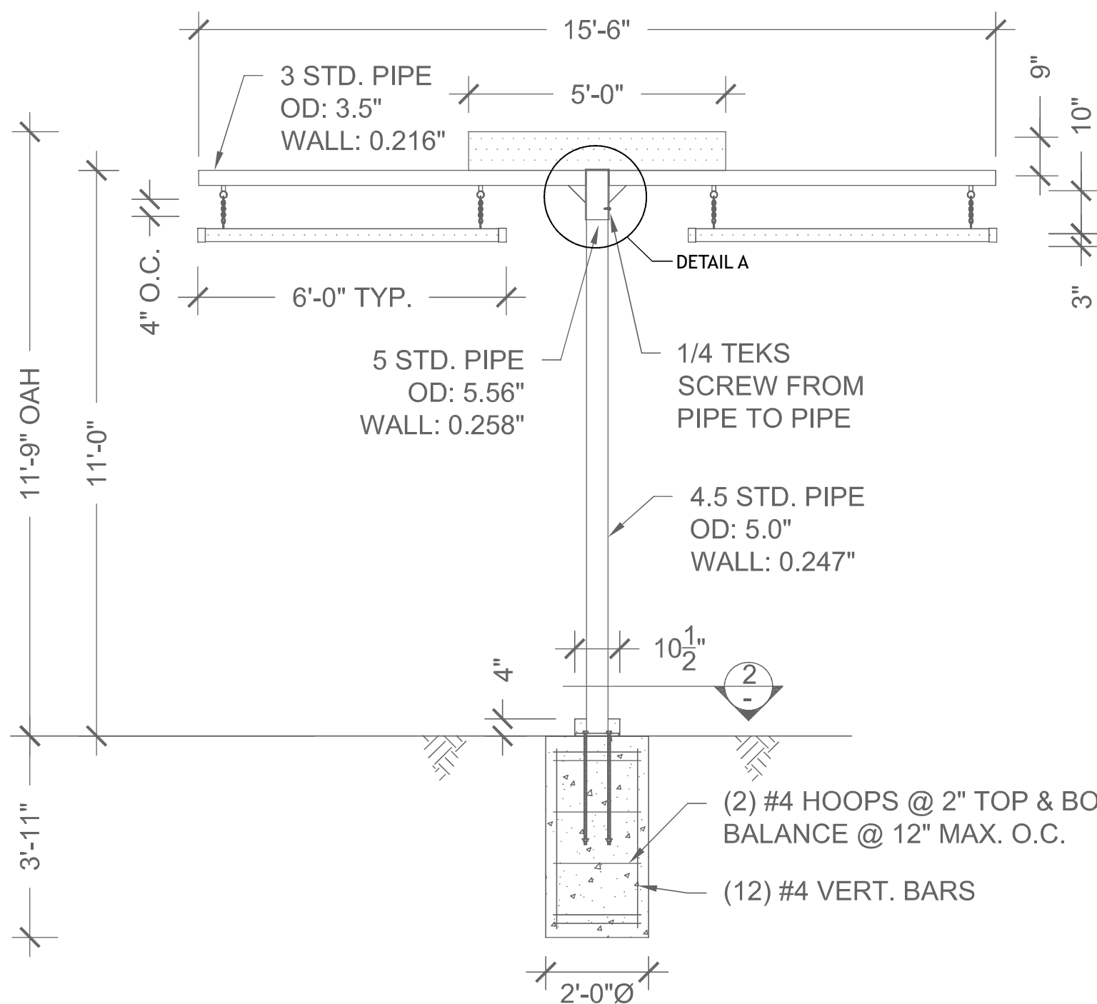
ELEVATION SCALE: 3/8" = 1'-0"
