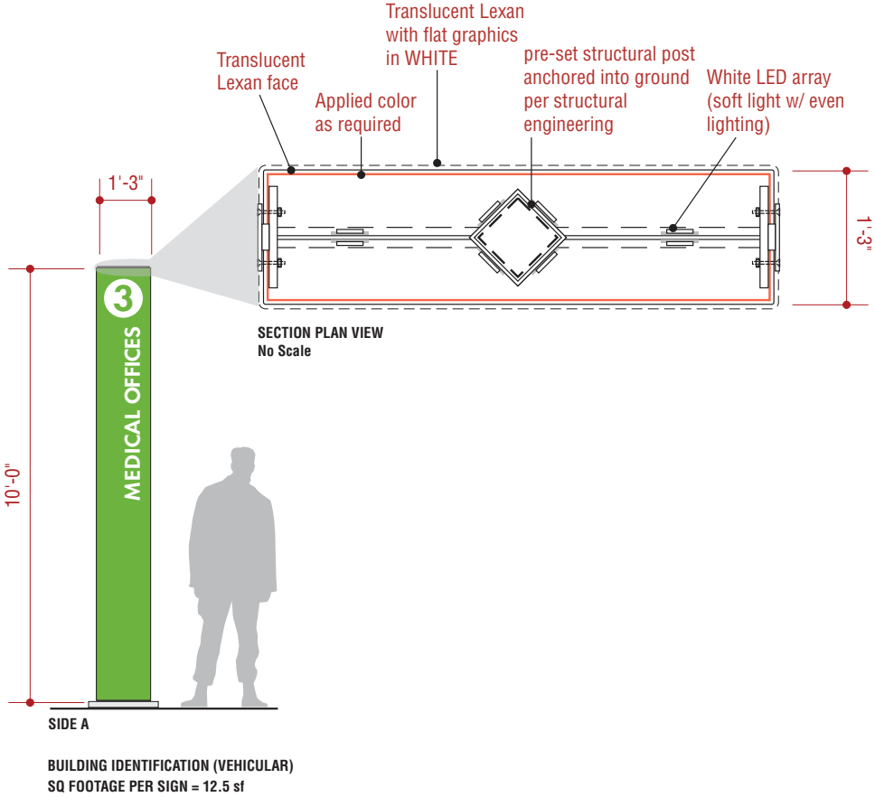
2 DETAIL LOC. 12.1 Scale: 1/4" = 1'-0"
