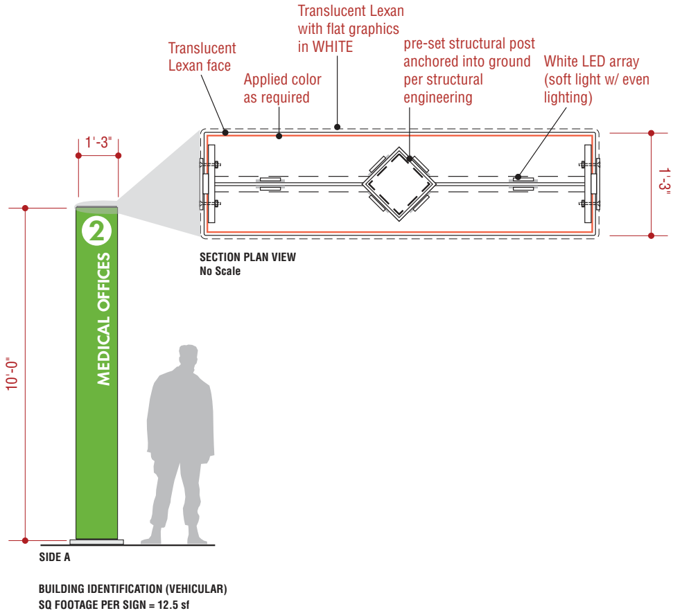
2 DETAIL LOC. 31.1 Scale: 1/4" = 1'-0"
