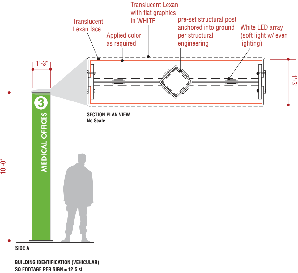
2 DETAIL LOC. 51.2 Scale: 1/4" = 1'-0"
