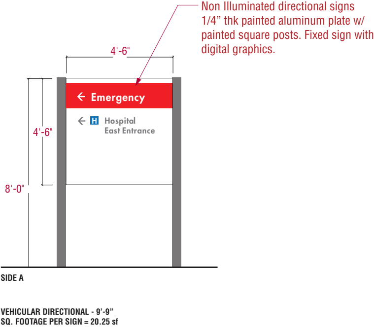
2 DETAIL LOC. 103 Scale: 1/4" = 1'-0"
