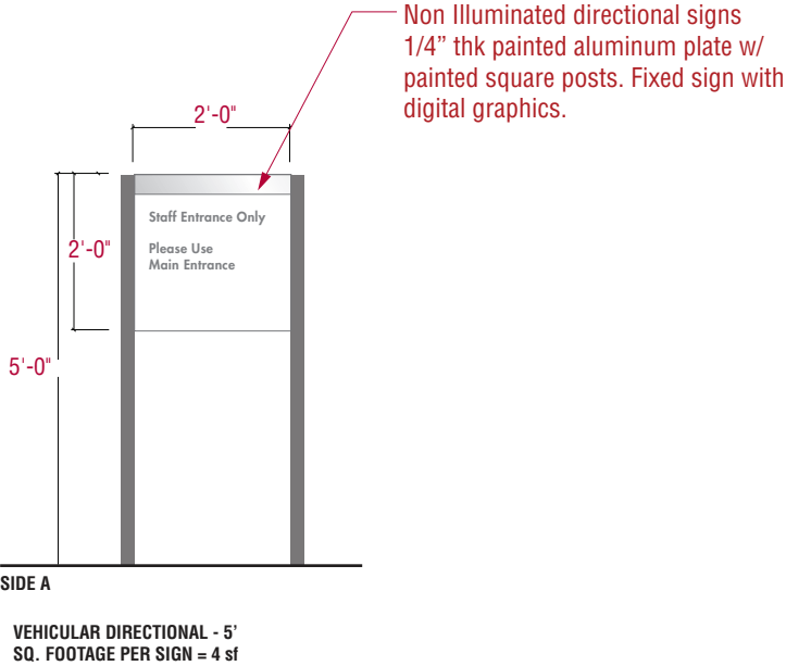
2 DETAIL LOC. 26 Scale: 3/8" = 1'-0"
