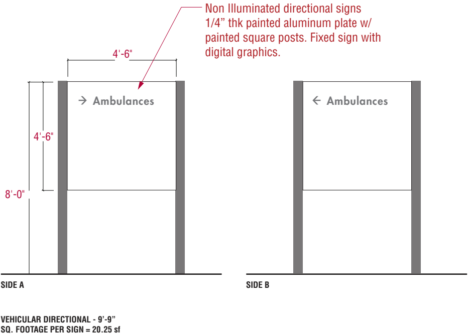
2 DETAIL LOC. 105 Scale: 1/4" = 1'-0"
