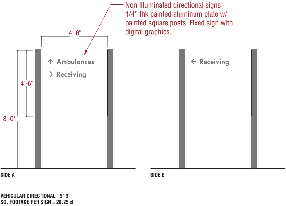
2 DETAIL LOC. 106 Scale: 1/4" = 1'-0"
