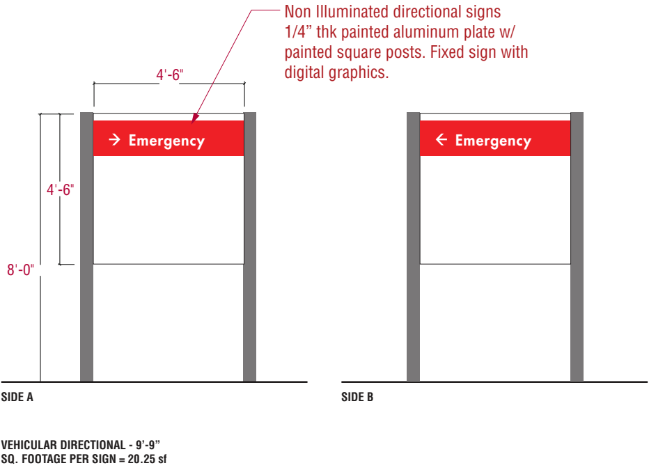
2 DETAIL LOC. 104 Scale: 1/4" = 1'-0"
