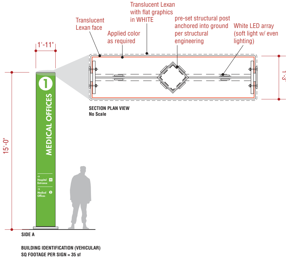
2 DETAIL LOC. 18.1 Scale: 3/16" = 1'-0"
